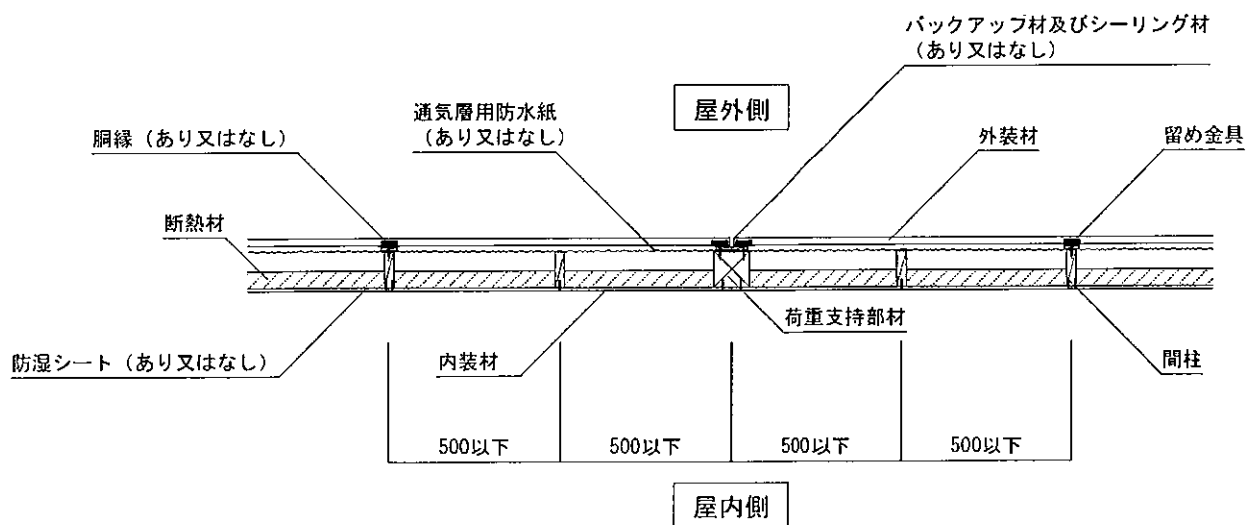
鉛直断面図
