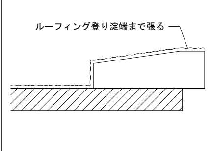
ルーフィング詳細図（縮尺1/3）
