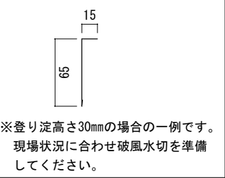
破風水切参考図（現場調達）
