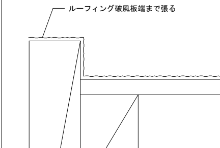
ルーフィング詳細図（縮尺1/3）
