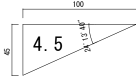
ルーフィング張り詳細図（縮尺：1/10）
