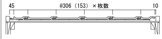
パターン② F 1 半瓦を使用しない場合（縮尺：1/25）※ 2
