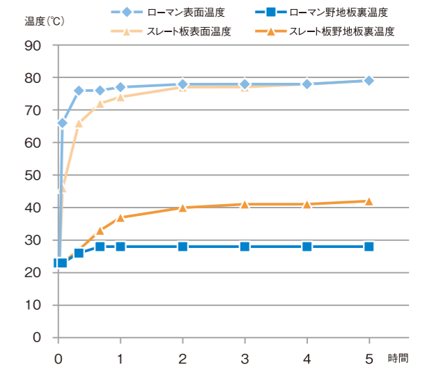
夏場の裏面温度 41℃
