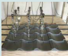
耐風圧性能試験
