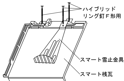
スマート雪止（角）
