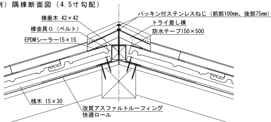
例) 隅棟断面図（4.5寸勾配）
