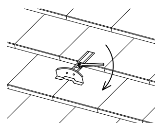
スパナ（13サイズ）又はレンチ トルク：122.4kgf・cm（12.5N・m）
