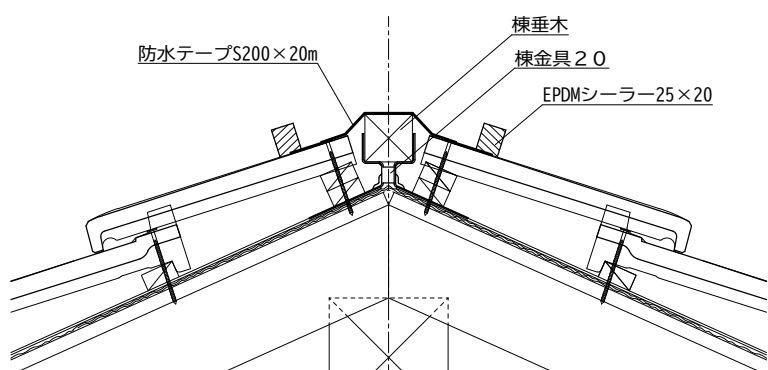
例) 大棟断面図 (4.5寸勾配)
