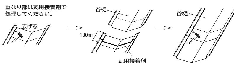
〔谷樋 重なり部〕
