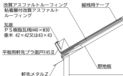
【角材の瓦座】（緩勾配は角材の瓦座を推奨）
