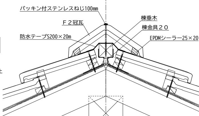
例) 大棟断面図 (4.5寸勾配)
