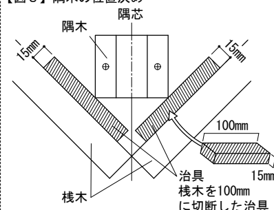
【図 3】隅木の位置決め
