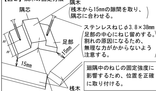
【図 2】隅木の固定方法
