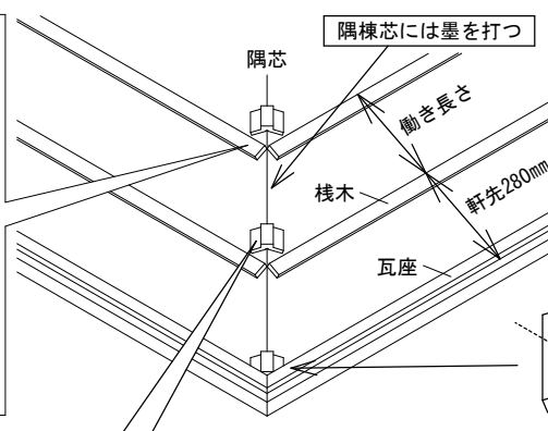
【図 3】隅木の位置決め
