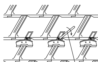
スパナ (13 サイズ) 又はレンチ トルク：122.4kgf・cm (12.5N・m)
