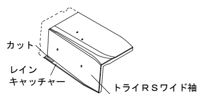
【棟際の棧瓦が半端物】
