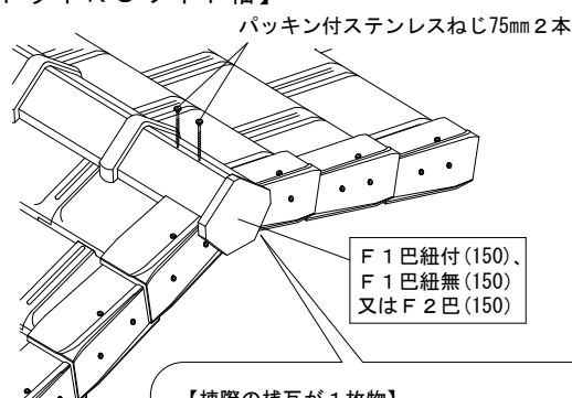
【棟際の棧瓦が1枚物】
