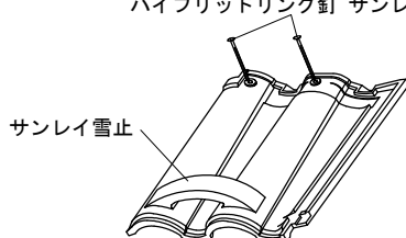
ハイブリッドリング釘 サンレイ用
