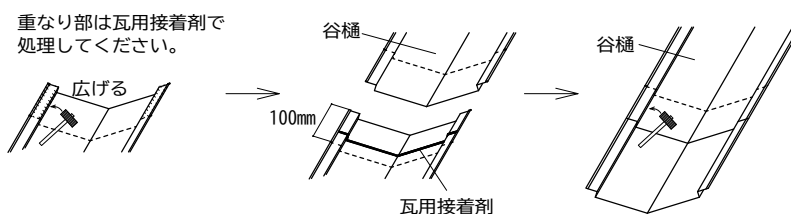
〔谷樋 重なり部〕
