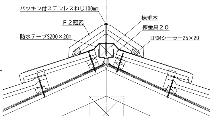
例) 大棟断面図 (4.5寸勾配)
