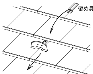
雪止金具本体部を手前に引き 瓦に止まっているか確認
